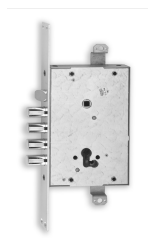
FIAM 672 GF, cyl. ISEO R7
